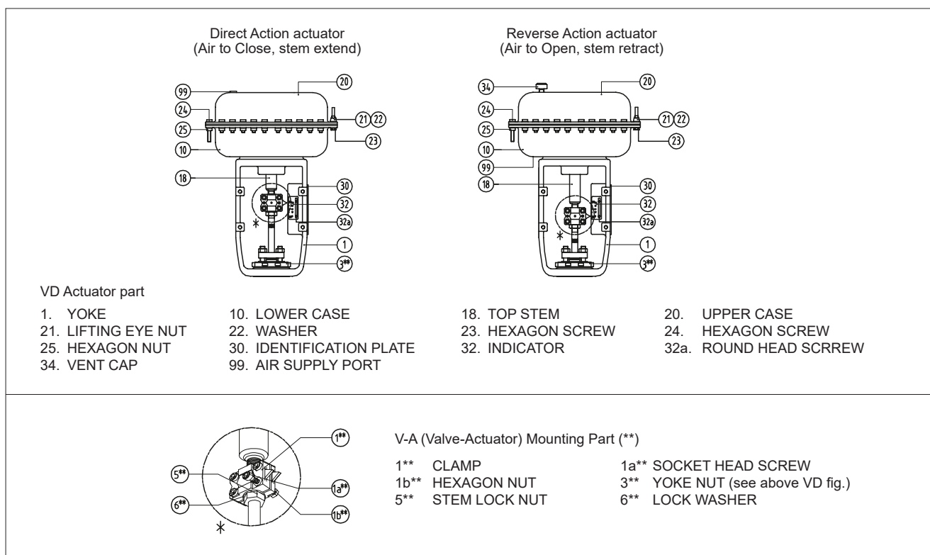
Fig. 14 VD Actuator
